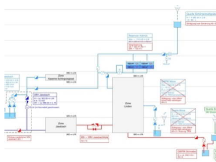
Hydraulisches Schema der Wasserversorgung mit Ausbaukonzept (in rot)
